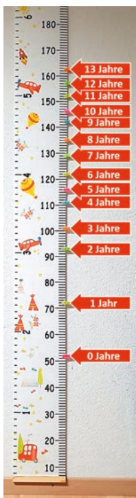
Abb. 1: Funktionaler Zusammenhang im Kinderzimmer: Eintragen der Körpergrößen auf der Messlatte
