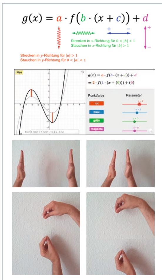
Abb. 5: Auswirkung von Parametern auf Funktionsgraphen
